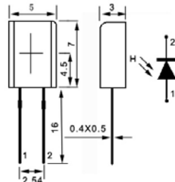
外形尺寸 (mm) 及内部电路示意图
